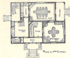
Fig. 4. Hoels plan.
